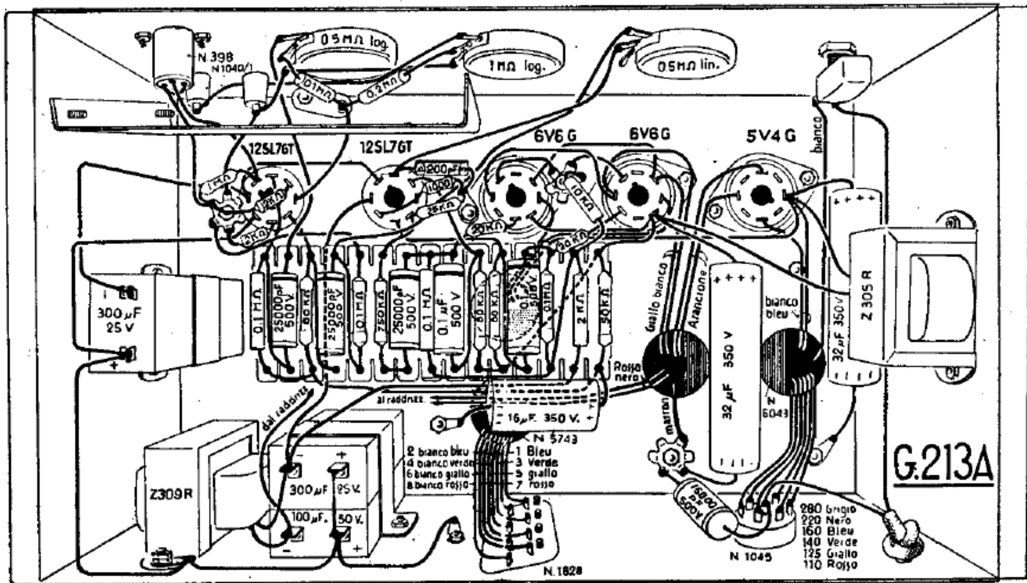
Lo schema costruttivo.
